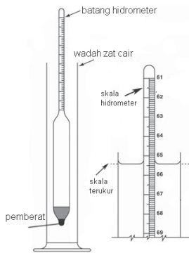
Gambar 7.10 Hidrometer
