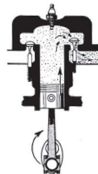
Gambar 9.12 Gerak pembuangan
