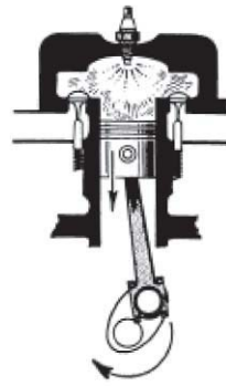
Gambar 9.11 Gerak tenaga
